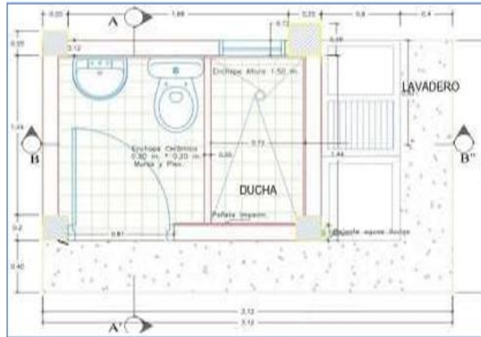
Plano planta Unidas Sanitaria
